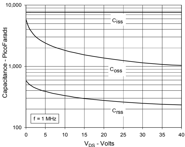
Fig. 11. Capacitance
